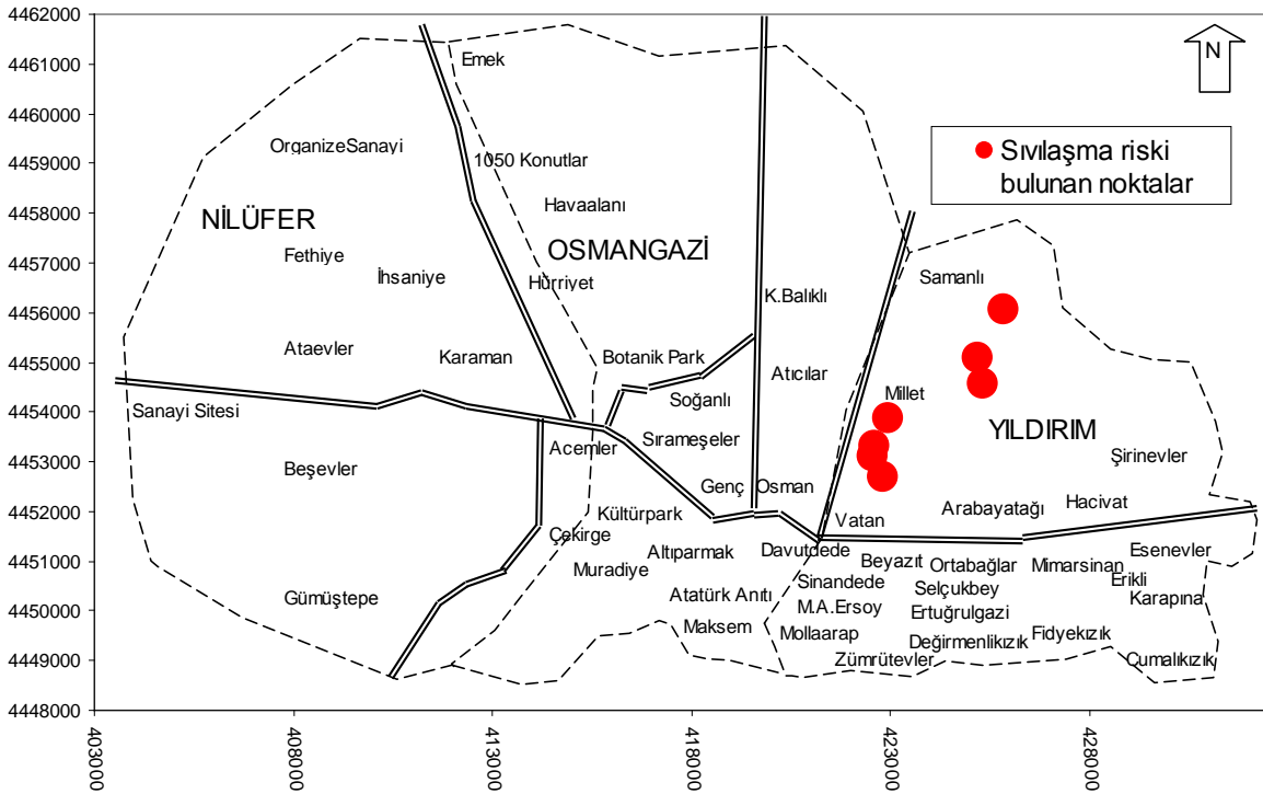
Şekil 7. Yüzey ivmesi 0.4g ve magnitüdü 7.5 olan bir deprem için sıvılaşma riski tespit edilen noktalar
