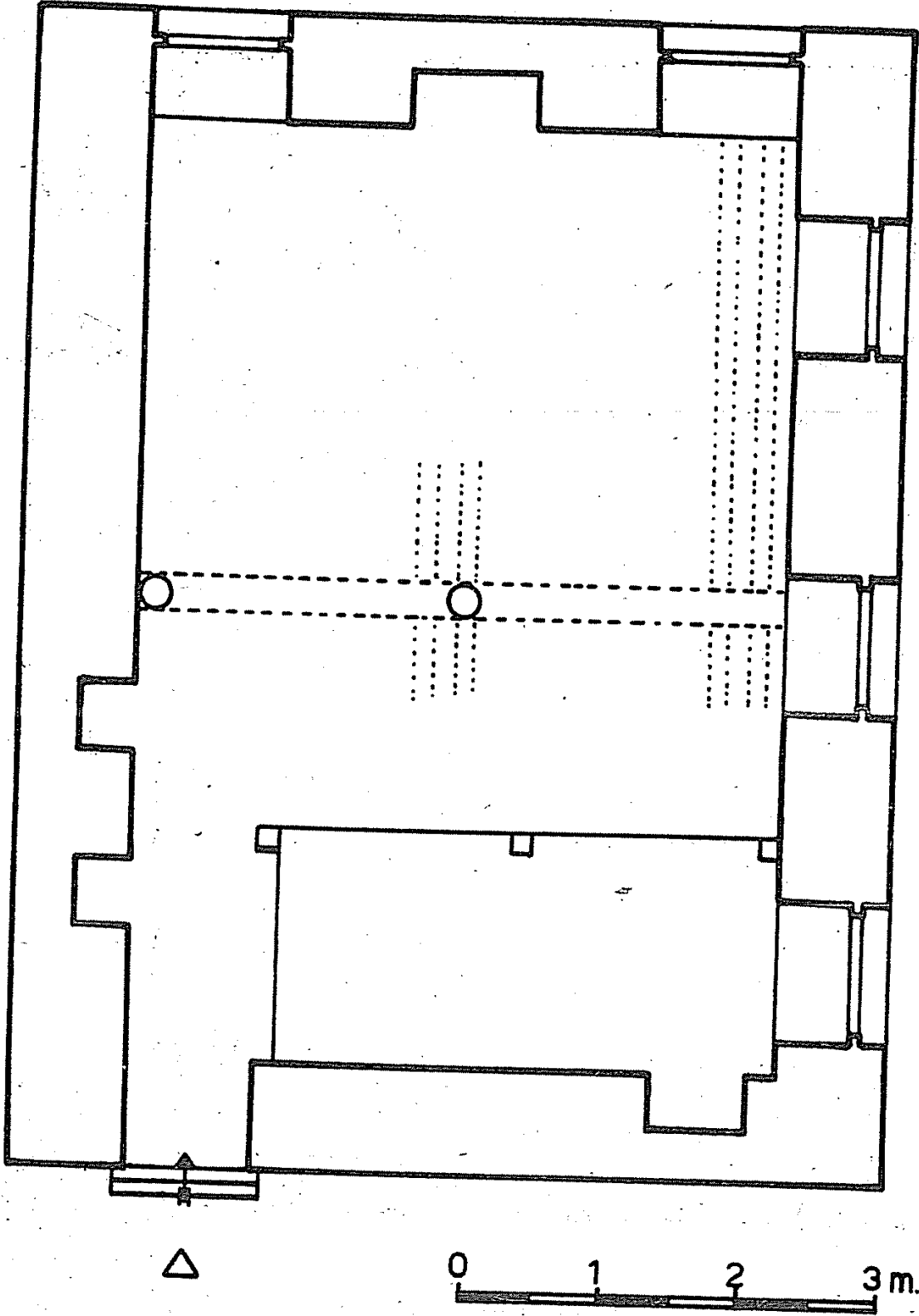
4. Şekil: Kamerolu (Taşbaşı) Mescidi Planı
