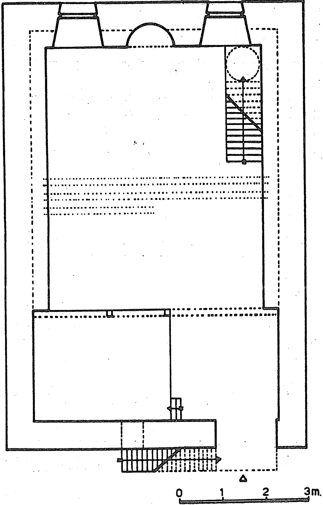
1. Şekil: Tekke Mescidi Plânı
