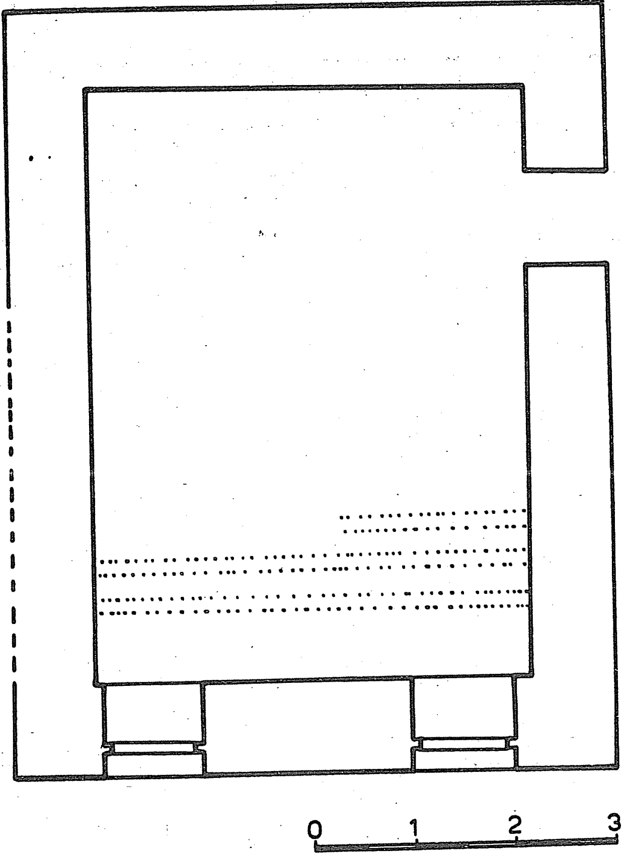
3. Şekil: Latif Ağa Mescidi Alt Kat Plânı
